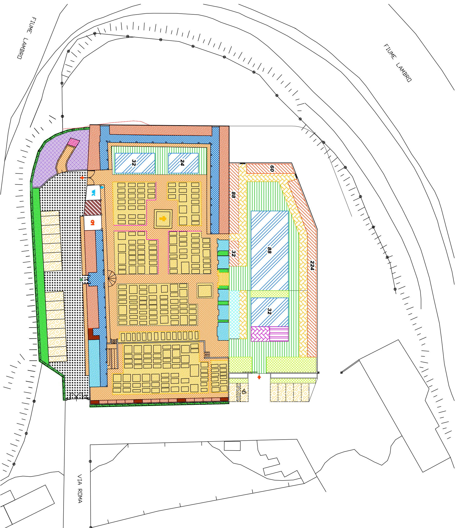
PLANIMETRIA STATO DI PROGETTO (scala 1:200)
